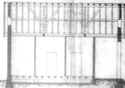
Corte Longitudinal.
