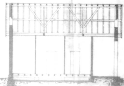
Corte Longitudinal.
