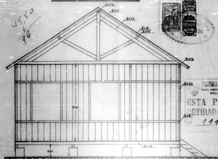
CORTE TRANS. 1:50
