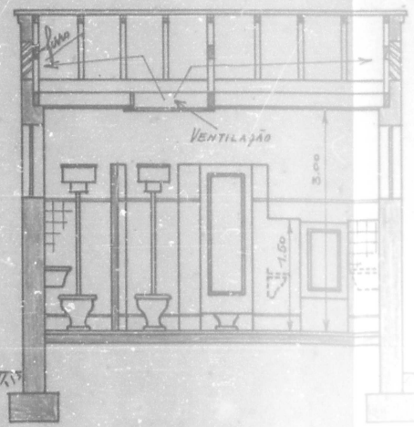
CORTES 1:50
