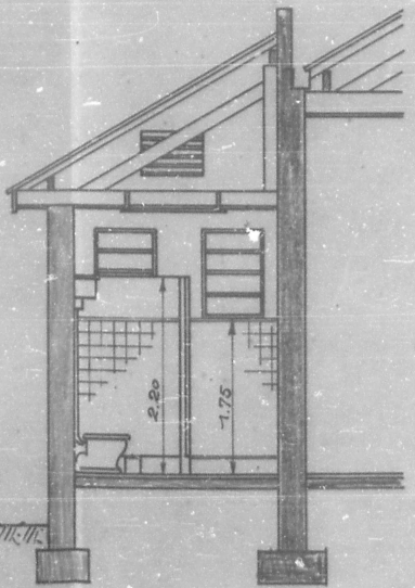
CORTES 1:50
