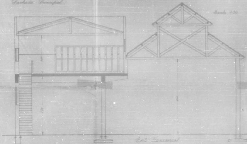
Corte Transversal
