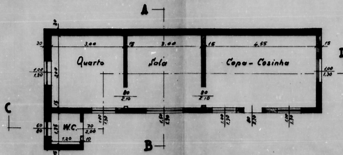
PLANTA
