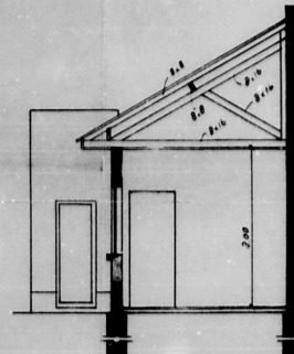
CORTA "AB"
