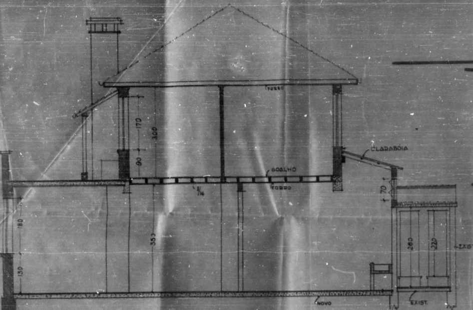
CORTE - C.D.
