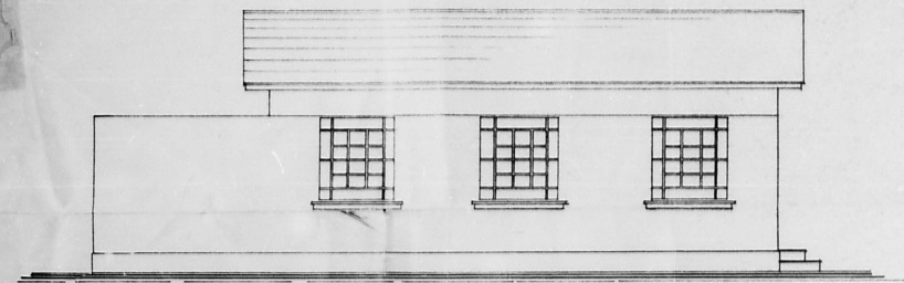
- FACHADA - 1:50 -
