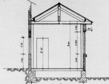
- CORTE TRANSVERSAL - 1:50 -
