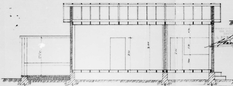
- CORTE LONGITUDINAL - 1:50 -
